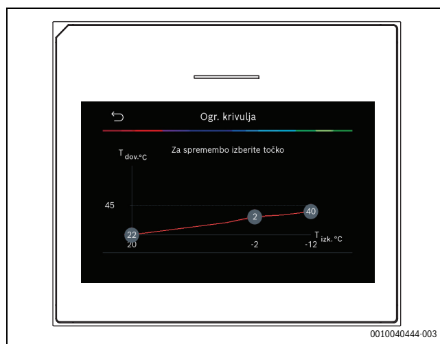
Obr. 1 Úvodná obrazovka na nastavenie vykurovacej krivky pre typ regulácie vonkajšej teploty pomocou päťm bodu (a komfortného bodu)
