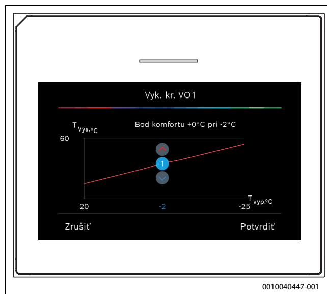
Obr. 4 Nastavenie komfortného bodu (iba ak je typ regulácie nastavený na vonkajšiu teplotu s päťm bodom)
