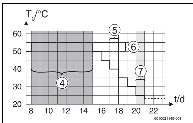
Obr. 8 Proces sušenia potu so základnými nastaveniami vo fáze chladenia
