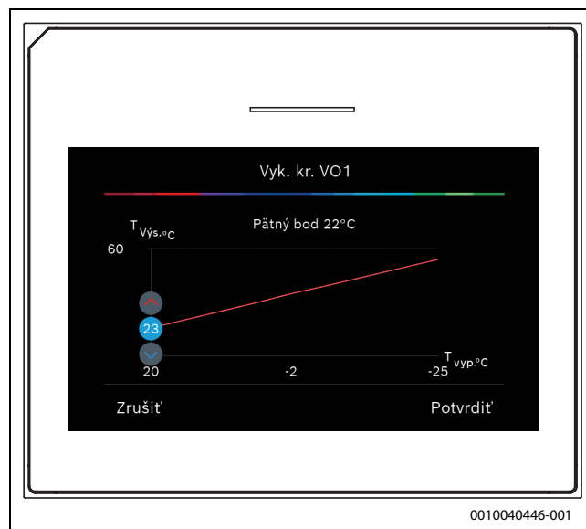
Obr. 3 Nastavenie päťm bodu (iba ak je typ regulácie nastavený na vonkajšiu teplotu s päťm bodom)
