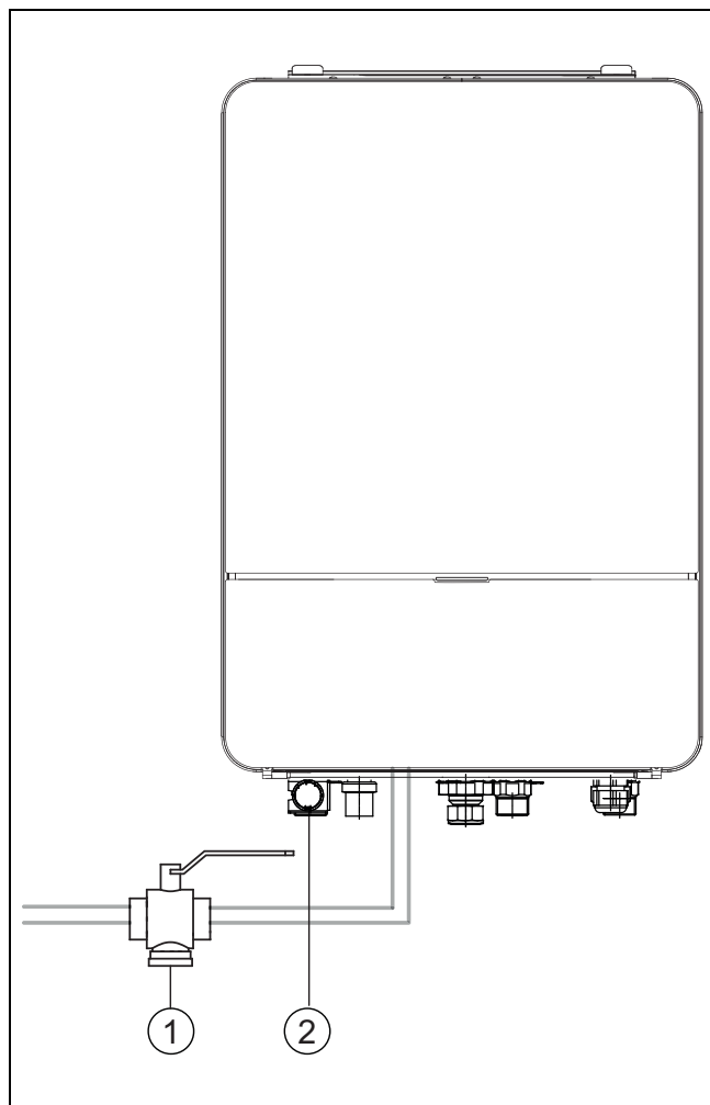
Obr. 7 Vnútrotná jednotka AWE
