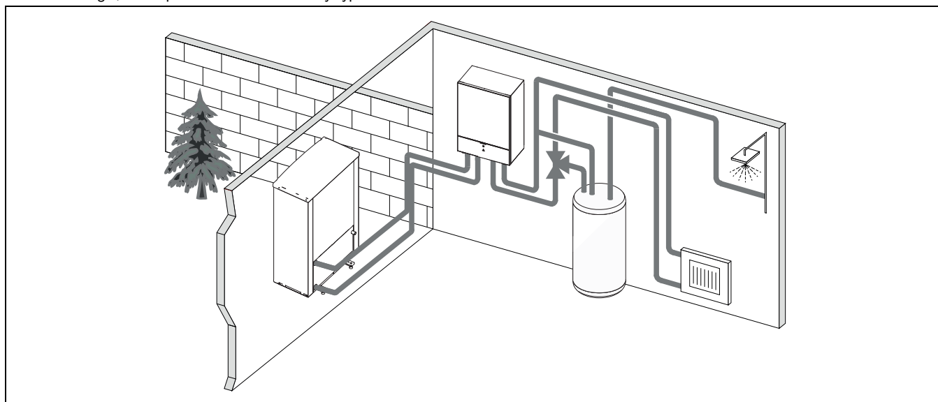
Obr. 3 Tepelné čerpadlo Compress 7000i AW, vnútoraná jednotka AWE s elektrickou vložkou pre dohrev a externým zásobníkom teplej vody
