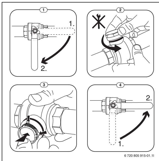
Obr. 8 Čistenie sitka
