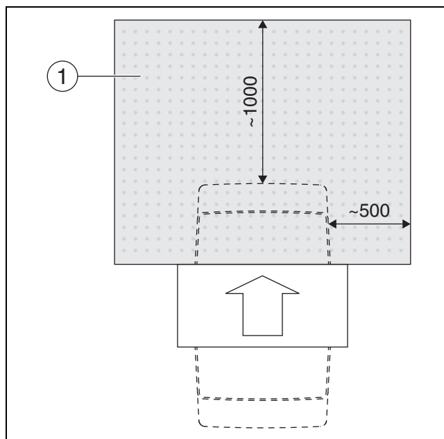
Obr. 11 NEBEZPEČENSTVO! Vytváranie ľadu pred tepelnými čerpadlami s protihlukovými krytmi (príslušenstvo)
