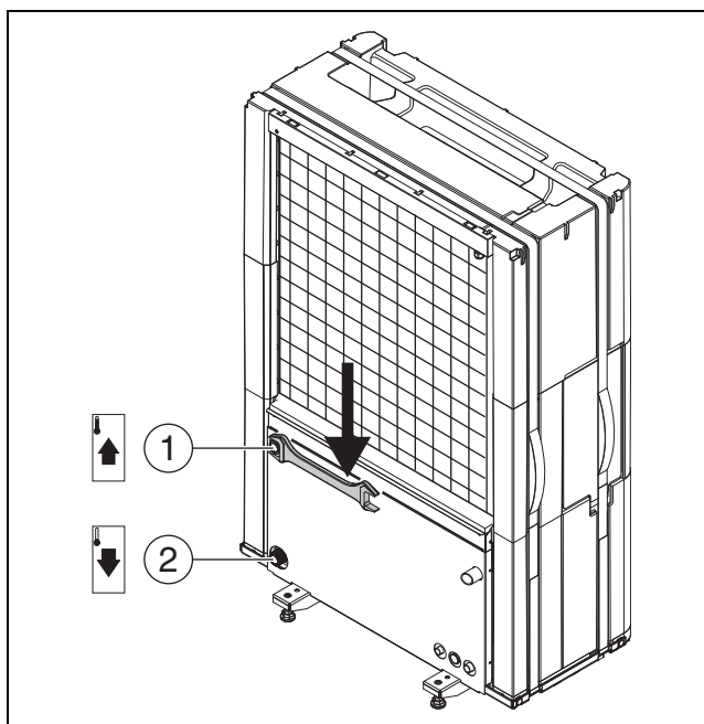
Obr. 18 Prípojky potrubí teplotného média, platí pre všetky veľkosti
