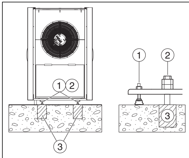
Obr. 14 Upevnenie tepelného čerpadla
