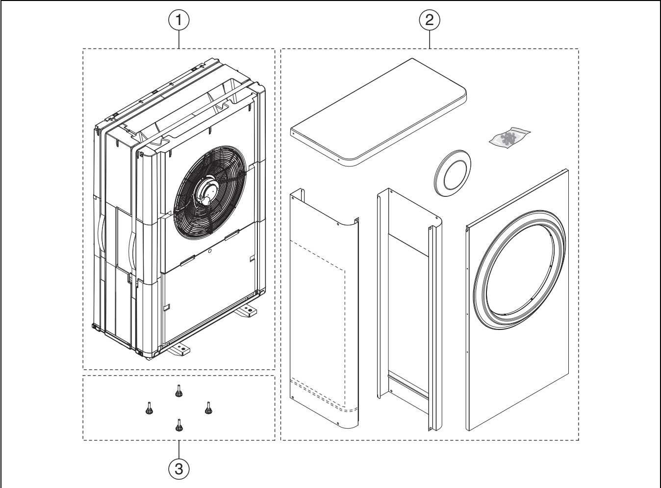
Obr. 2 Rozsah dodávky
