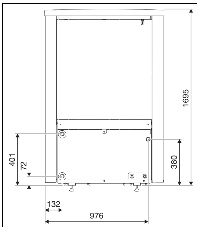
Obr. 6 Rozmery a prípojky modelov tepelného čerpadla 13 OR-T-17 OR-T, zadná strana
