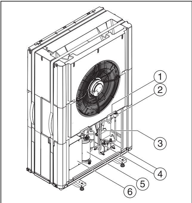
Obr. 3 Prehľad zariadenia
