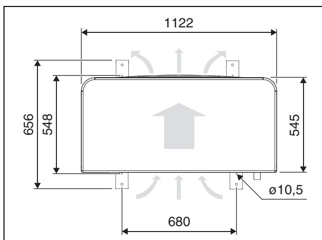
Obr. 7 Rozmery modelov tepelného čerpadla 13 OR-T-17 OR-T, pohľad zhora
