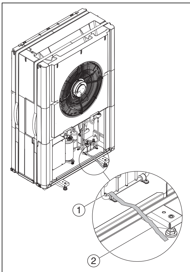
Obr. 13 Prepravná poistka
