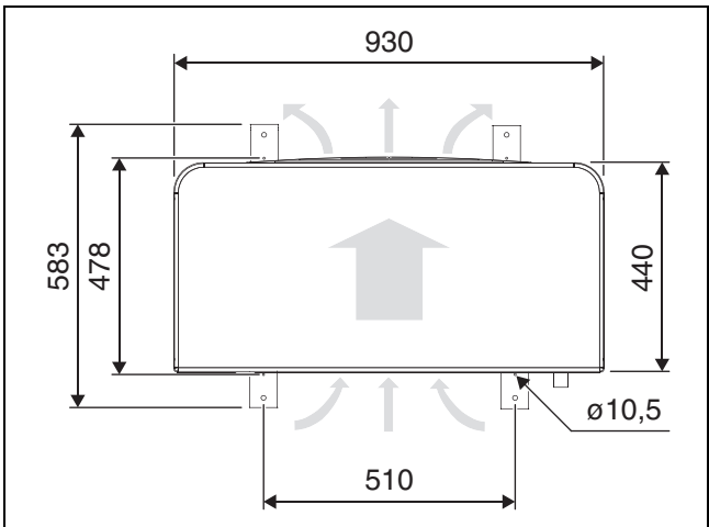
Obr. 5 Rozmery modelov tepelného čerpadla 5 OR-S-9 OR-S, pohľad zhora
