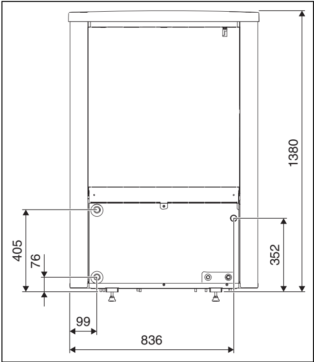
Obr. 4 Rozmery a prípojky modelov tepelného čerpadla 5 OR-S-9 OR-S, zadná strana
