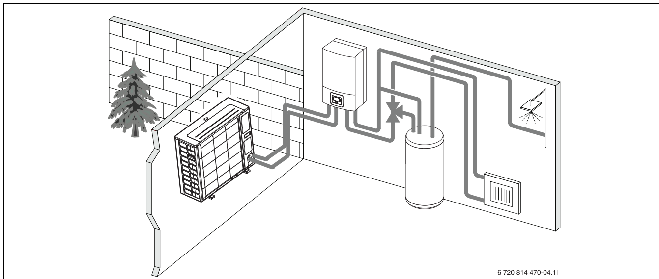
Obr. 2 Tepelné čerpadlo s vonkajšou jednotkou, vnútornou jednotkou AWES s elektrickou vložkou dohrevu a zásobníkom teplej vody
