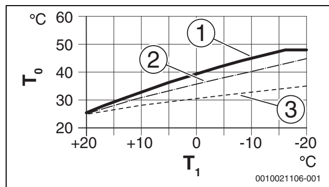
Obr. 2 Nastavenie vykurovacej krivky podlahového vykurovania Stúpanie pomocou dimenzačnej teploty T 0 a minimálnej vonkajšej teploty T 1,min
