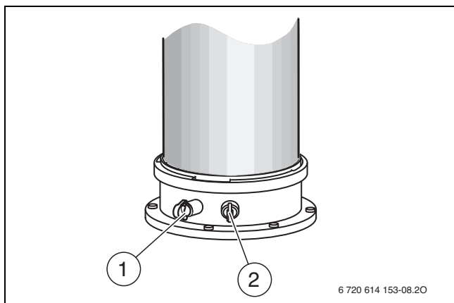
Obr. 52 Meracie hrdlo spalín a meracie hrdlo spaľovacieho vzduchu
