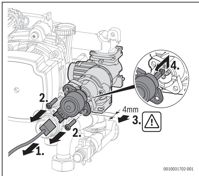
Obr. 84 Demontáž motora na 3-cestnom ventile (verzia so skrutkami)
