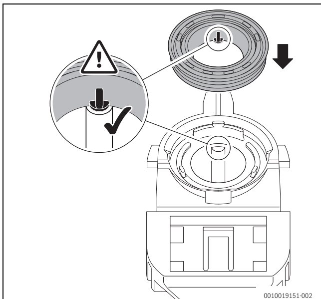
Obr. 69 Vyrovnanie nového tesnenia na sifóne na kondenzát
