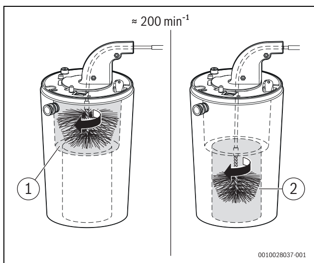
Obr. 63 Čistenie tepelného bloku (cca 200 \text{ min}^{-1} , len v smere hodinových ručičiek)
