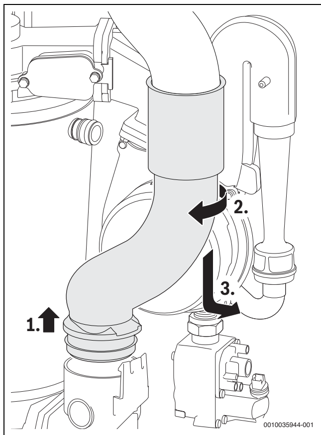
Obr. 54 Demontáž rúry pre odvod spalín
