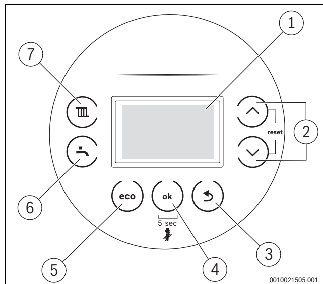
Obr. 44 Ovládacie pole
