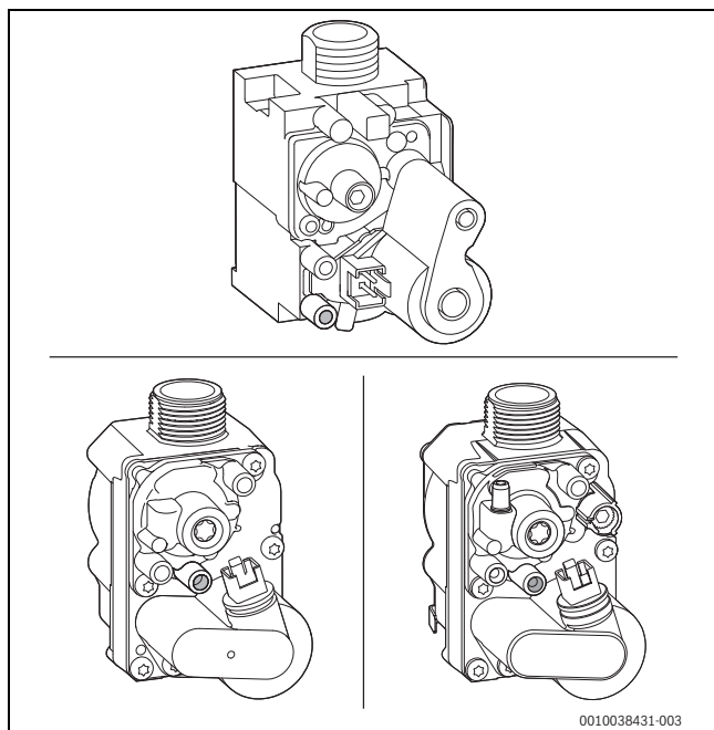
Obr. 46 Vľavo hore a dole: nenastaviteľná plynová armatúra, vpravo dole: nastaviteľná plynová armatúra
