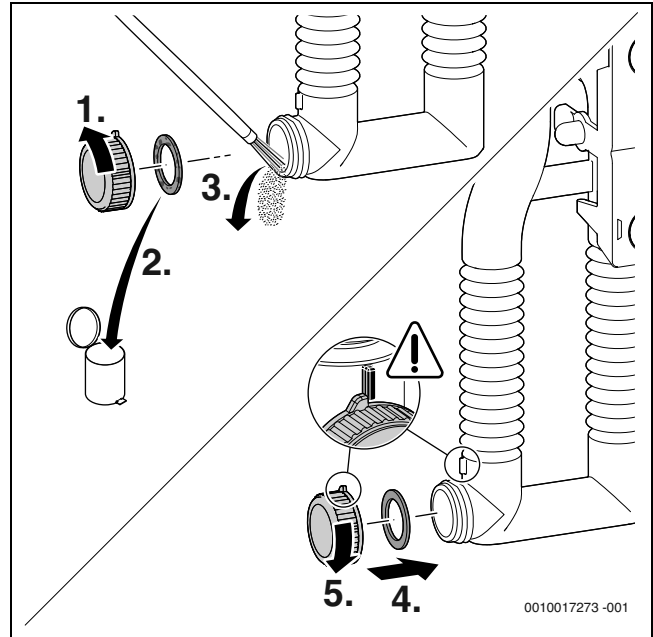
Obr. 67 Čistenie sifónu na kondenzát
