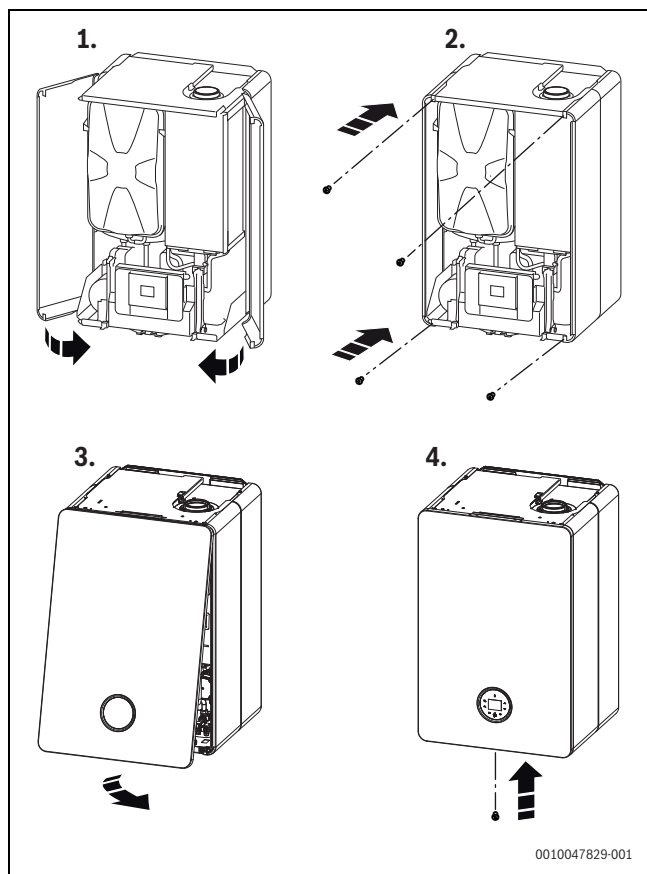
Obr. 43 Montáž plášťa
