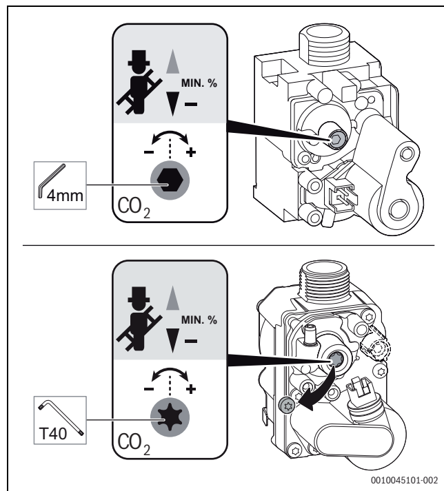
Obr. 51 Nastavenie obsahu CO 2 /O 2 pri minimálnom menovitom tepelnom výkone
