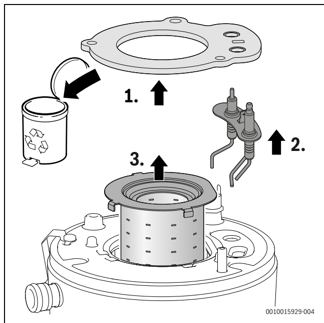
Obr. 58 Demontáž horáka
