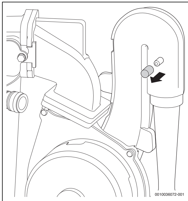
Obr. 53 Meracie hrdlo na zmiešavacom zariadení
