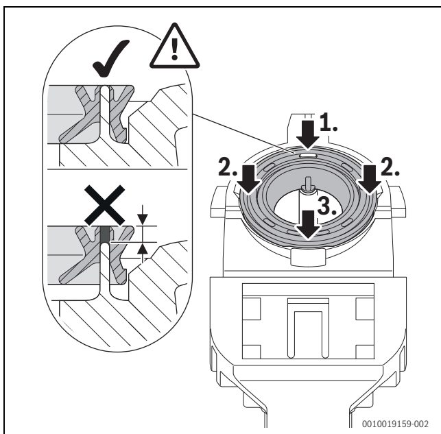
Obr. 70 Pritlačenie tesnenia
