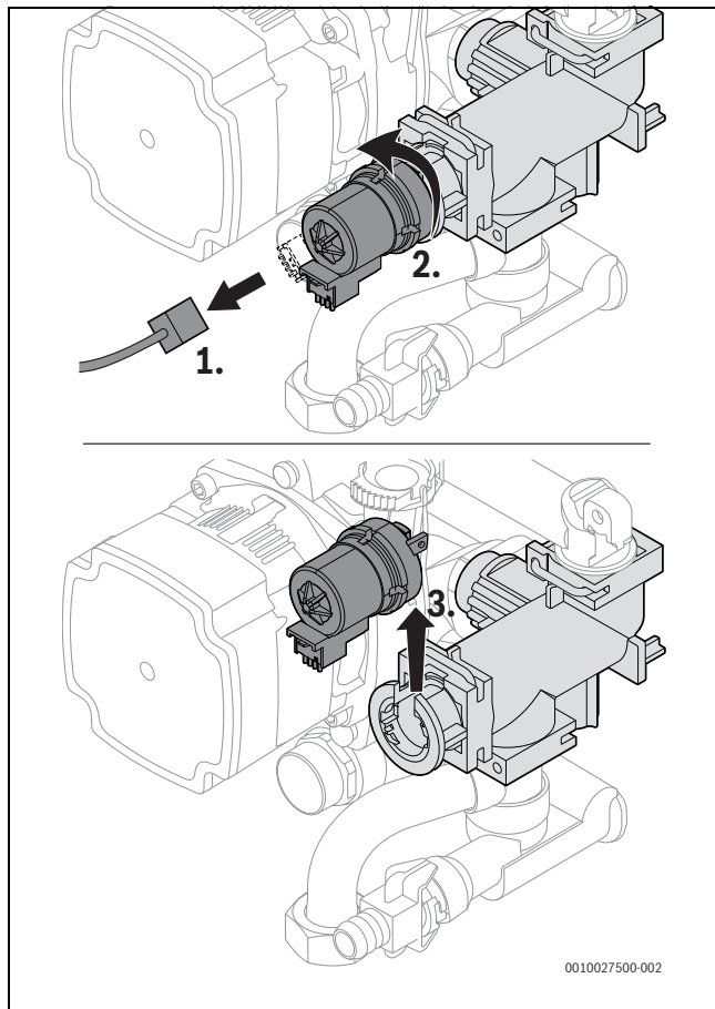
Obr. 82 Demontáž motora na 3-cestnom ventile (verzia bez skrutiek)
