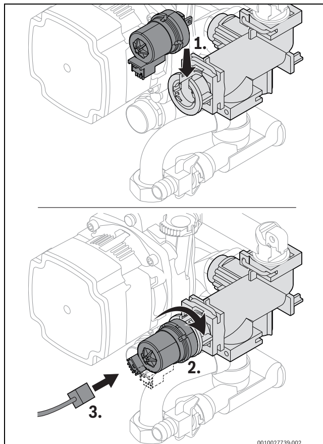
Obr. 83 Montáž motora na 3-cestnom ventile (verzia bez skrutiek)
