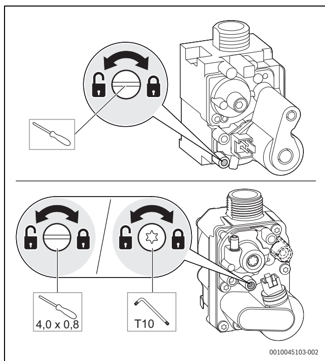
Obr. 48 Meranie pripojovacieho tlaku plynu
