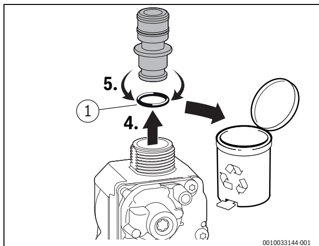
Obr. 75 Vybratie škrtiacej klapky plynu
