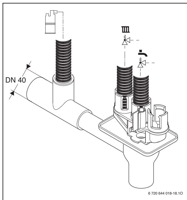
Obr. 35 Montáž hadice kondenzátu a hadice poistných ventilov na sifón
