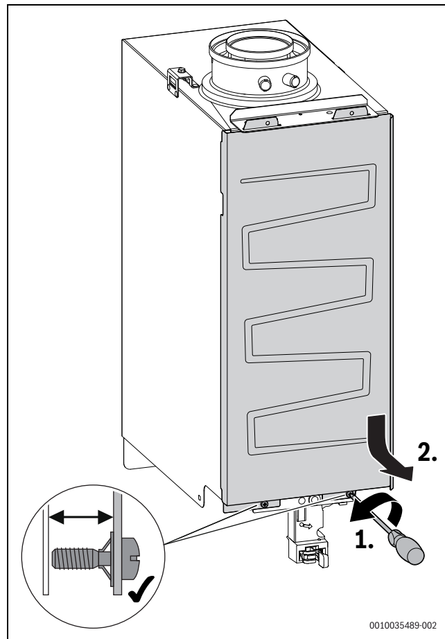
Obr. 47 Demontáž krytu horáka
