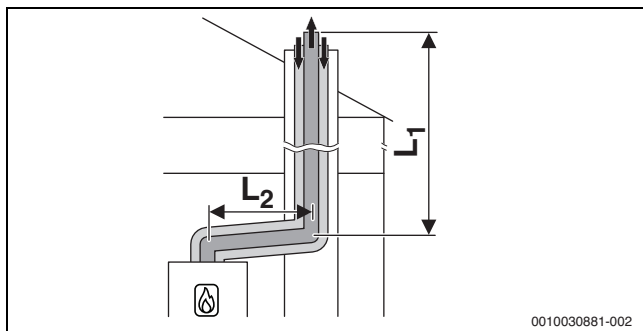
Obr. 9 Koncentrické vedenie vzduchu a spalín podľa C 33x v šachte
