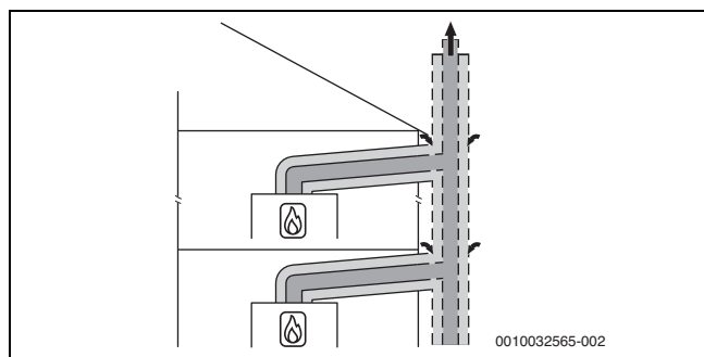
Obr. 20 Viacnásobné pripojenie podľa C (12)3x pomocou koncentrického vedenia vzduchu a spalín v miestnosti inštalácie
