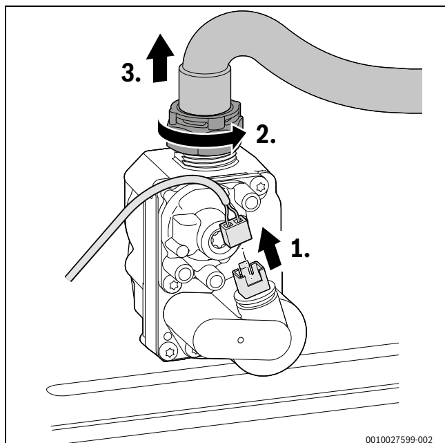
Obr. 74 Vytiahnutie zástrčky z plynovej armatúry a vybratie prevlečnej matice s plynovou hadicou
