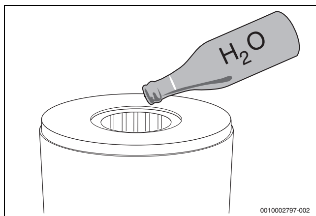
Obr. 65 Prepláchnutie tepelného bloku vodou
