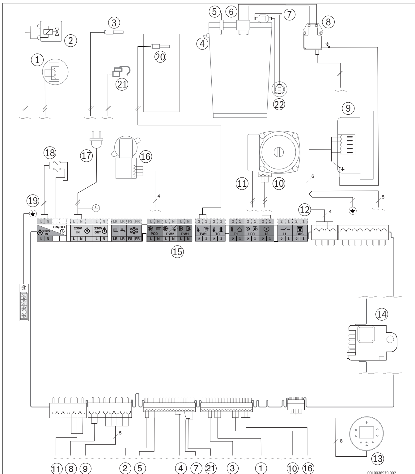
Obr. 87 Elektrické prepojenie vodičmi
