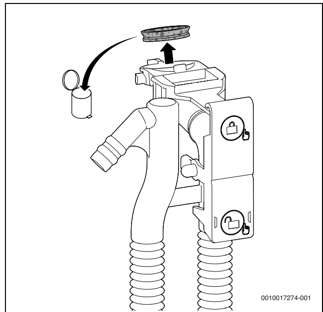
Obr. 68 Demontáž tesnenia v hornej časti sifónu na kondenzát
