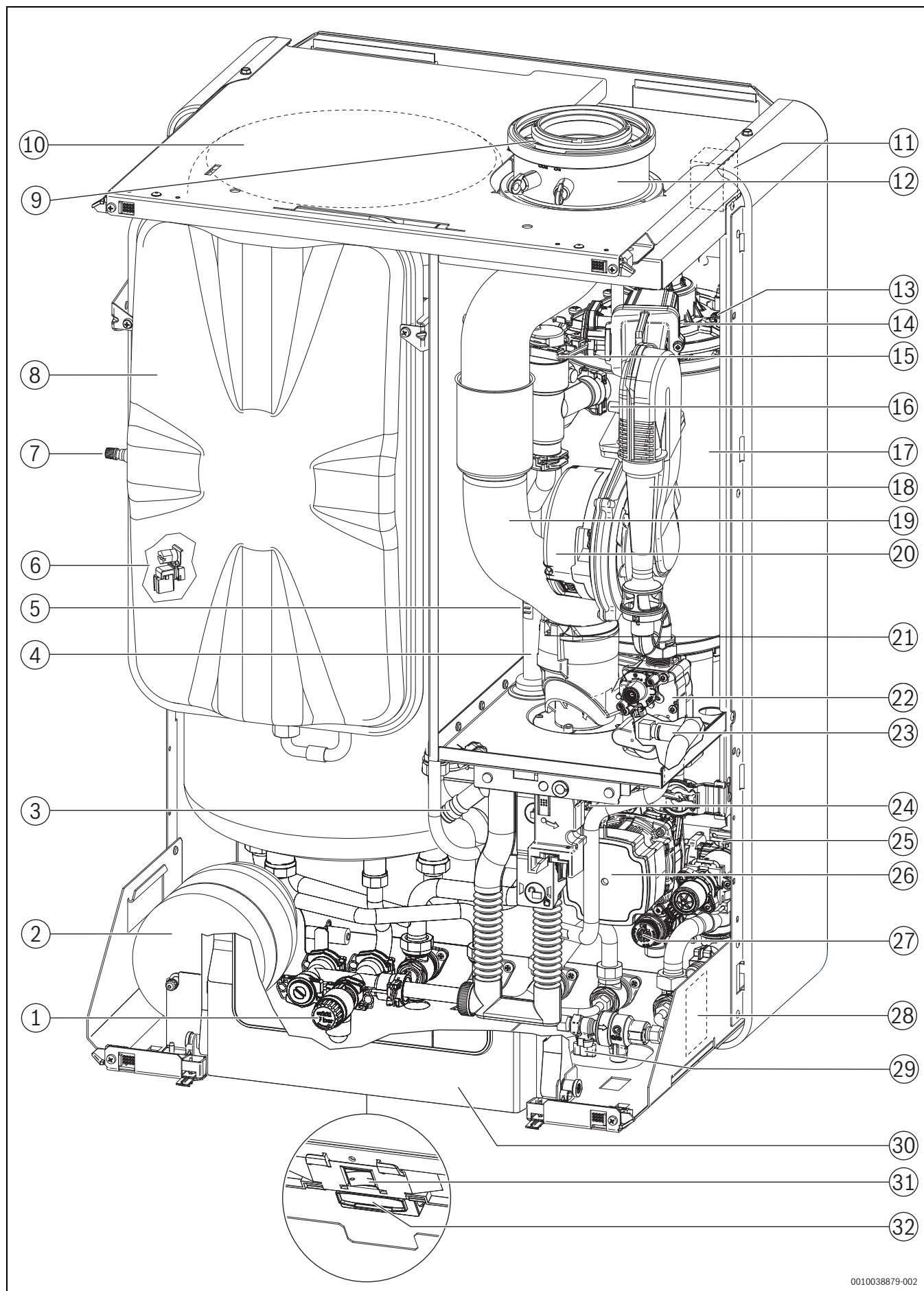
Obr. 5 Prehľad zariadenia
