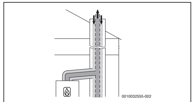
Obr. 11 Koncentrické vedenie vzduchu a spalín podľa C 43x v miestnosti inštalácie
