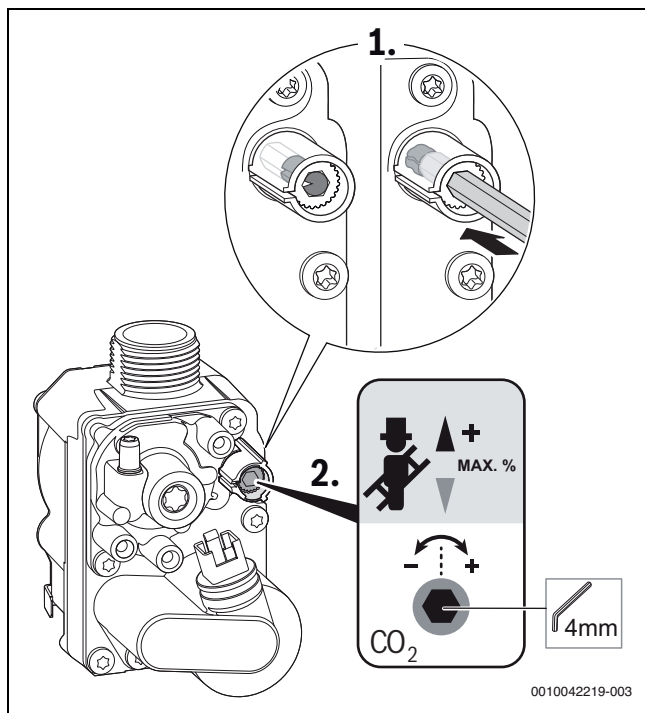
Obr. 50 Nastavenie obsahu CO 2 /O 2 pri maximálnom menovitom tepelnom výkone, nastaviteľná plynová armatúra
