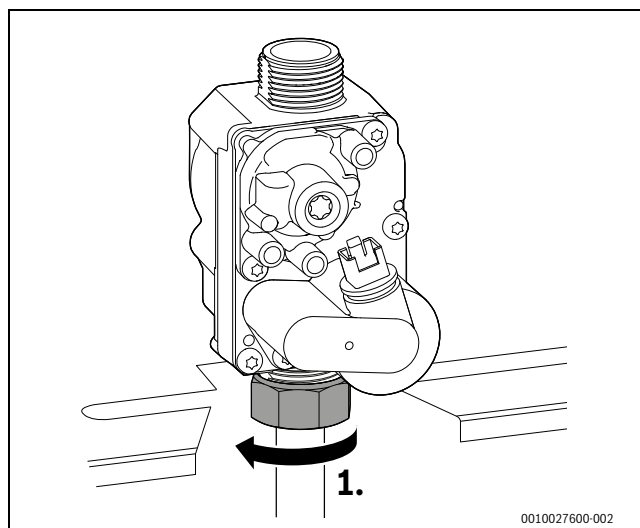
Obr. 76 Uvoľnenie prevlečnej matice
