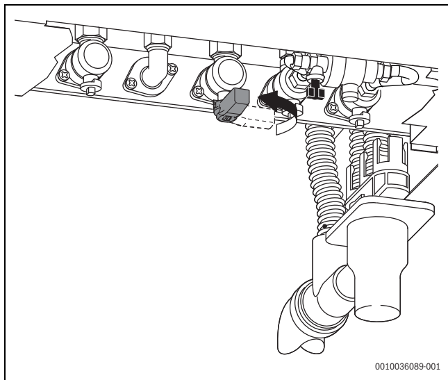
Obr. 5 Otvorenie plynového kohúta
