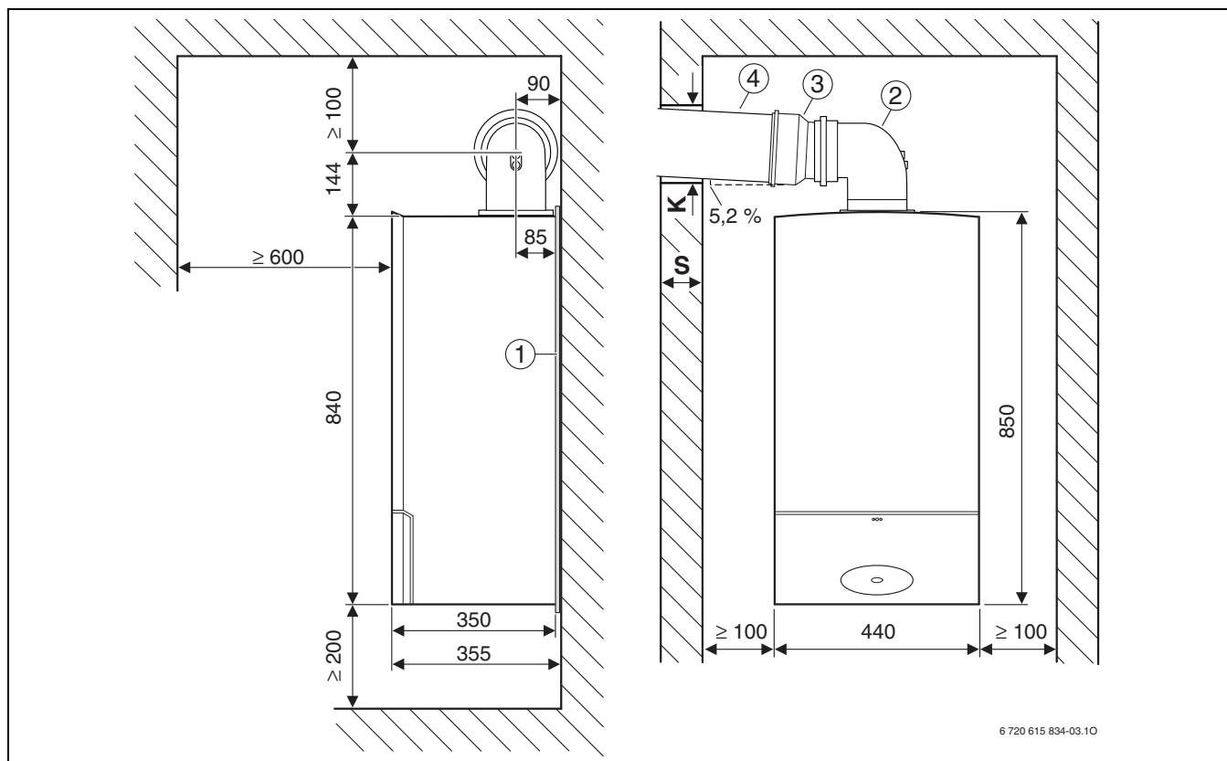
Obr. 7 Vedenie odvodu spalín Ø 100/150 mm
