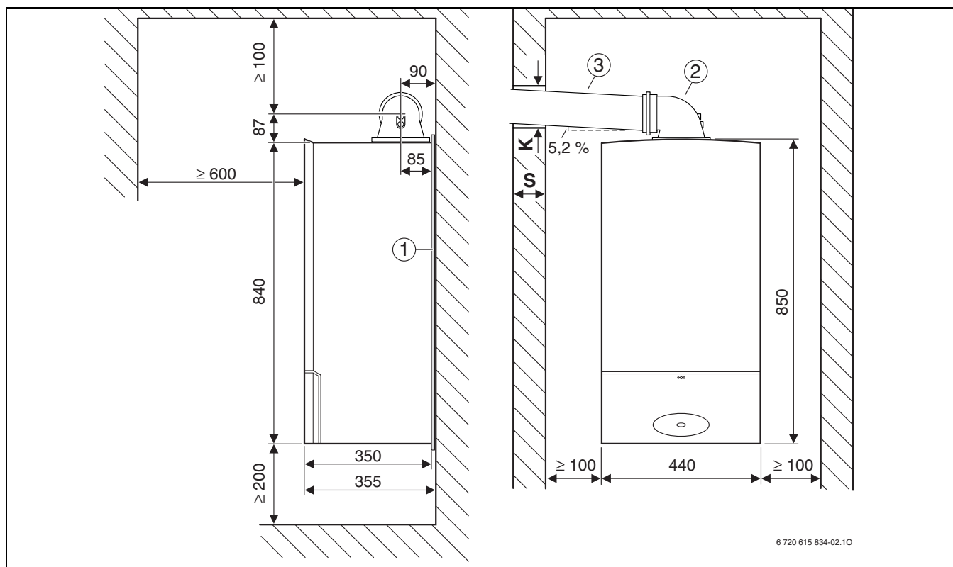
Obr. 6 Vedenie odvodu spalín Ø 60/100 mm
