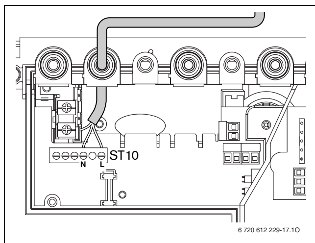
Obr. 30 Svorková lišta privodu napätia ST10
