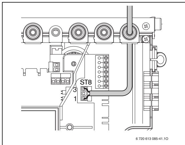
Obr. 25 Pripojenie termostatu zásobníka
