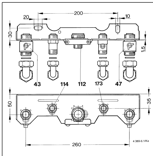
Obr. 9 Montážna pripojovacia doska (vertikálne pripojenie) č 492
