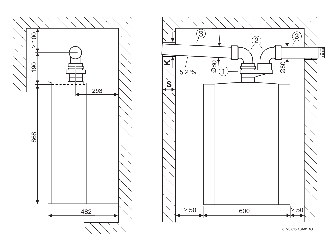
Obr. 9 Prívod vzduchu/odvod spalín v oddelených potrubíach (Ø80 mm)
